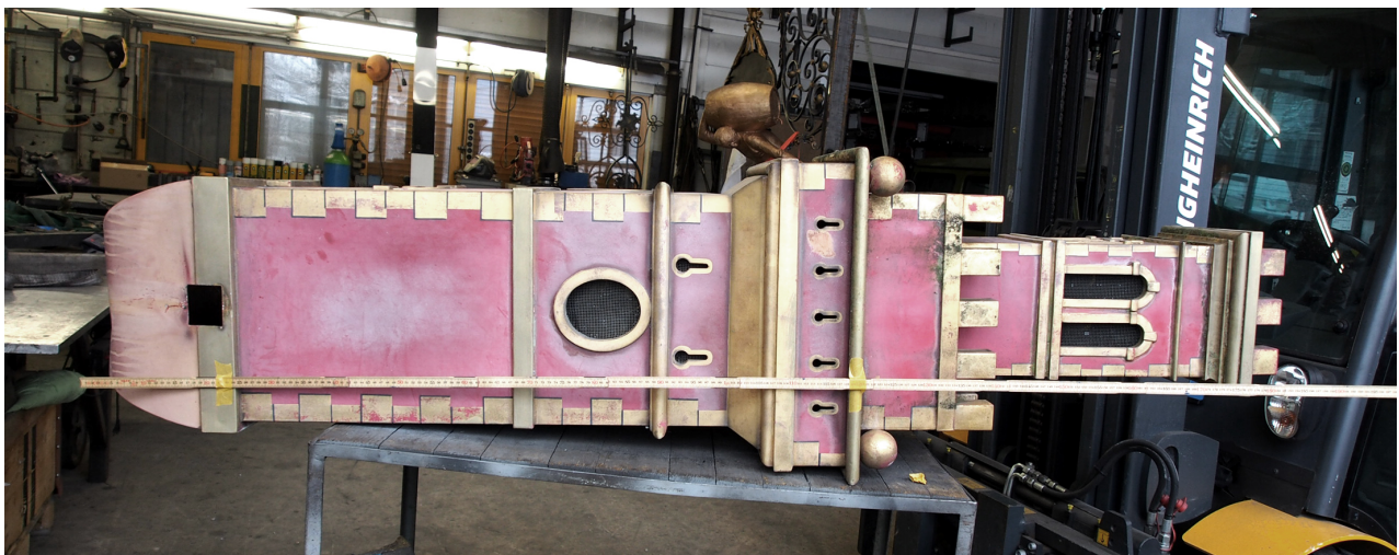
Abb.3: Demontiertes Türmchen in der Werkstatt von Toni Maccaferri, während der Vermassung für die Planaufnahme.
